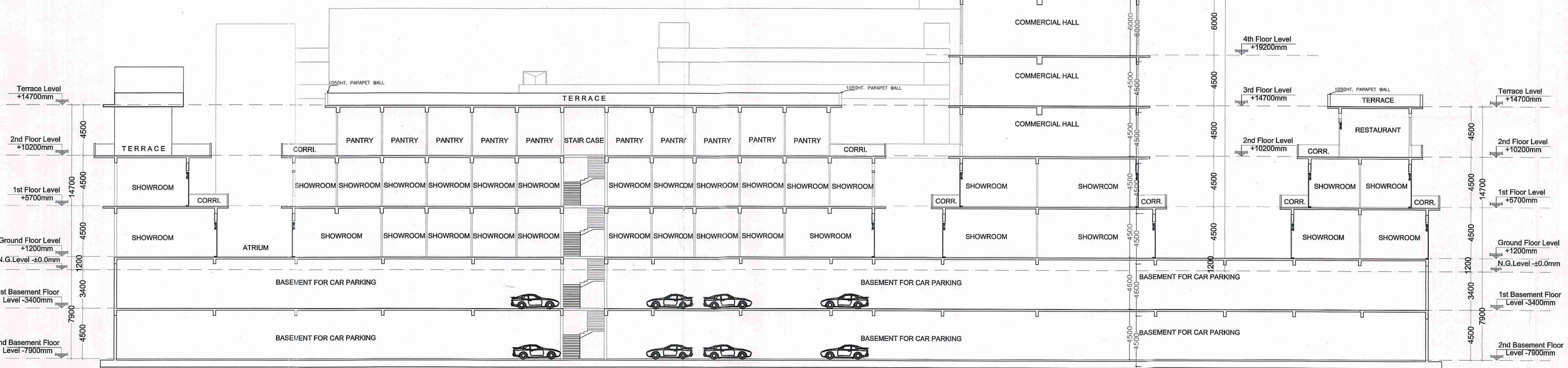
SECTION A-A
